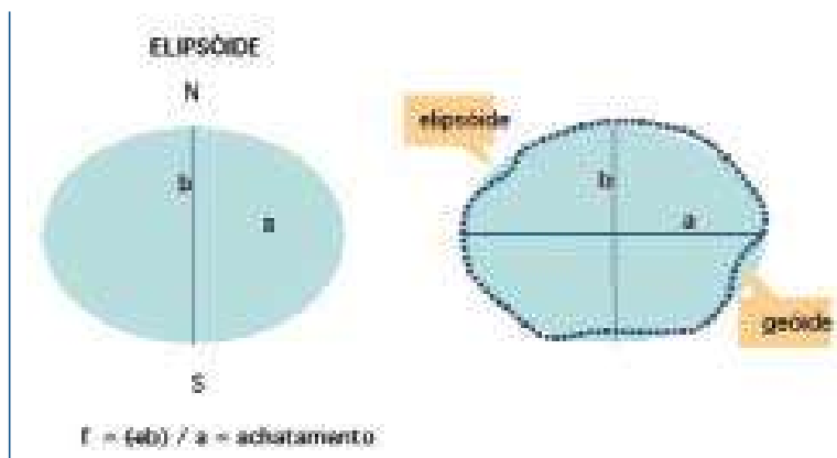
Figura 4: Representação do elipsóide e do geóide.
