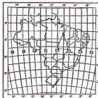
Figura 7: Fusos UTM sobre o Brasil (Fonte: IBGE, 1998)
